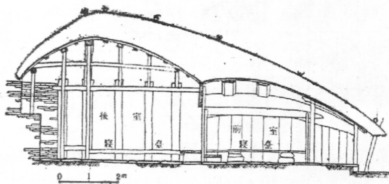
圖片說明：恆春上蕃外麻里巴力社 Ararai Baritiyo 家屋剖面圖
