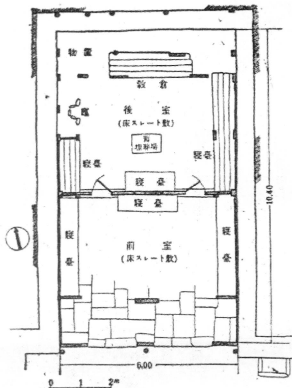
圖片說明：內文社恆春上蕃、外麻里巴力社 Ararai Baritiyo 家屋平面圖
