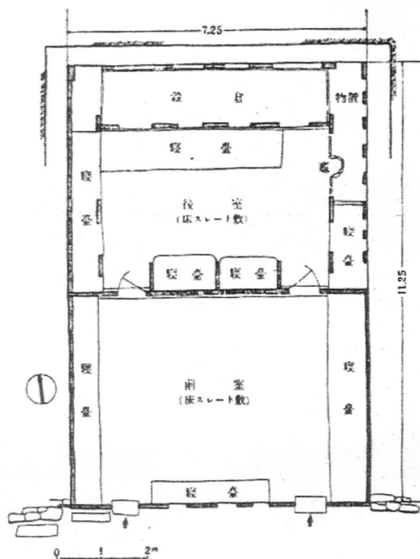
圖片說明：恆春上蕃ナイブン社 Robania Chujui 家屋平面圖
