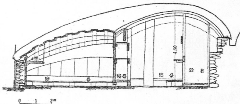
圖片說明：恆春上蕃ナイブン社 Robania Chujui 家屋剖面圖
