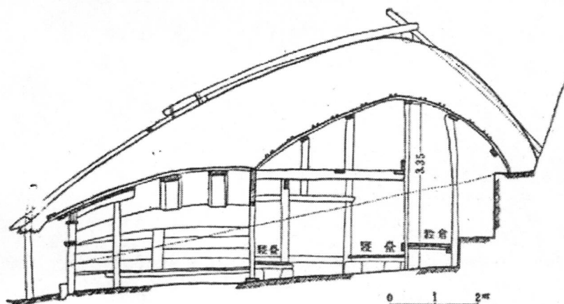
圖片說明：恆春下蕃ソウバウ社 Pabokku Chujui 家屋剖面圖
