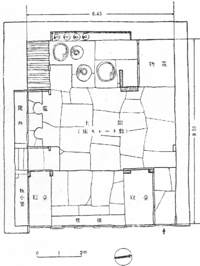
圖片說明：德文遺址家屋平面圖（千千岩, 1960：162）
