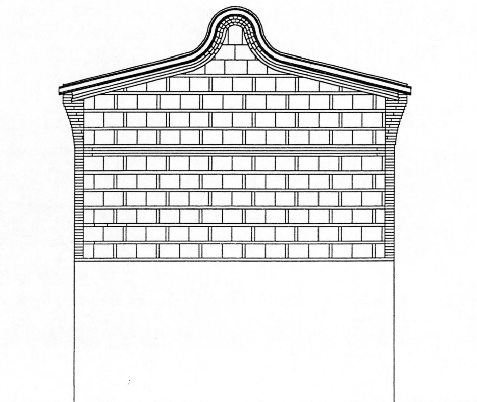
側立面圖
