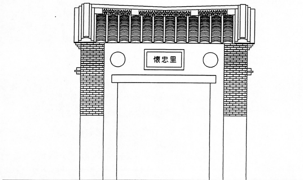
正向立面圖
