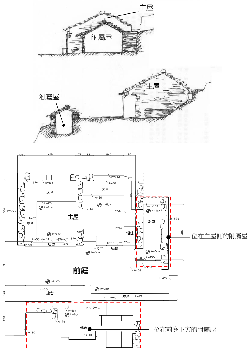
【圖 3-2-3】附屬屋與主屋關係配置圖 18
