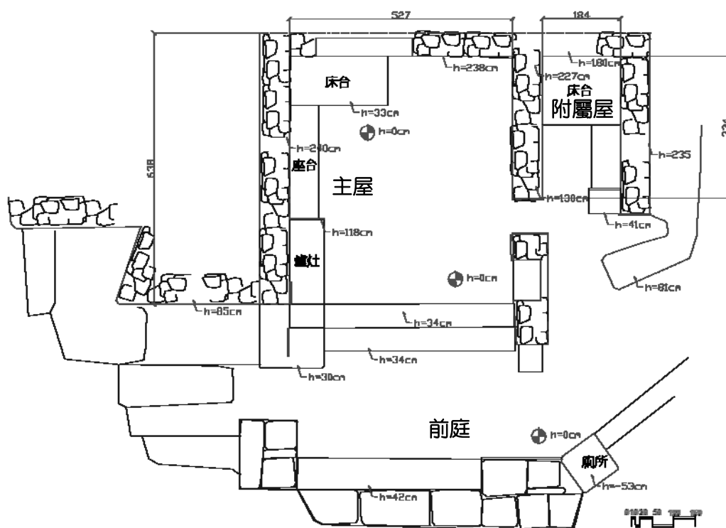
【圖 3-2-1】傳統家屋基本構成元素與配置 16
