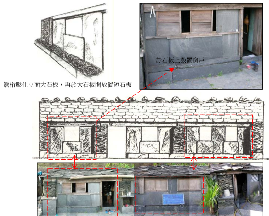
先放置二片大石板，中間再放置小石板，將窗戶圍塑出來(家屋編號 4 邱金士，2006)
