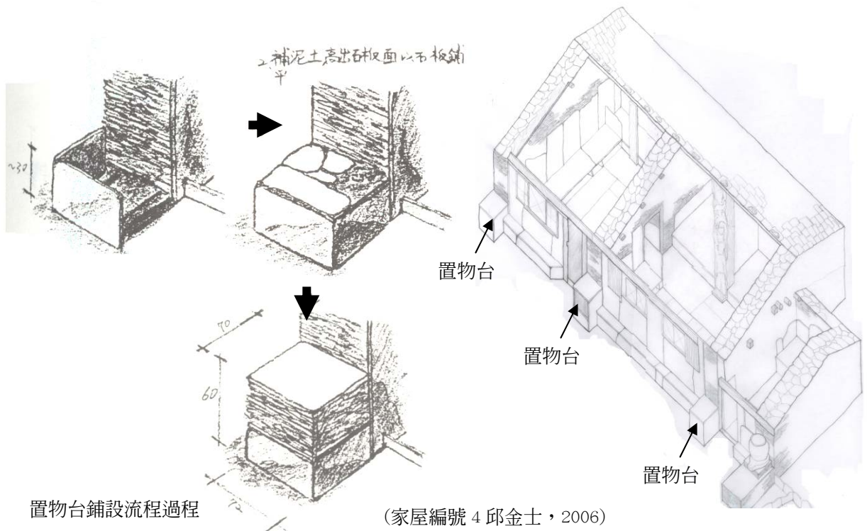
側牆前之置物台
