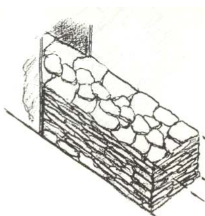
兩側放置較大石板，中間放置小石片之方式堆疊
