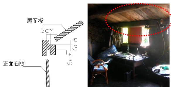
屋面板和簷桁的接法
