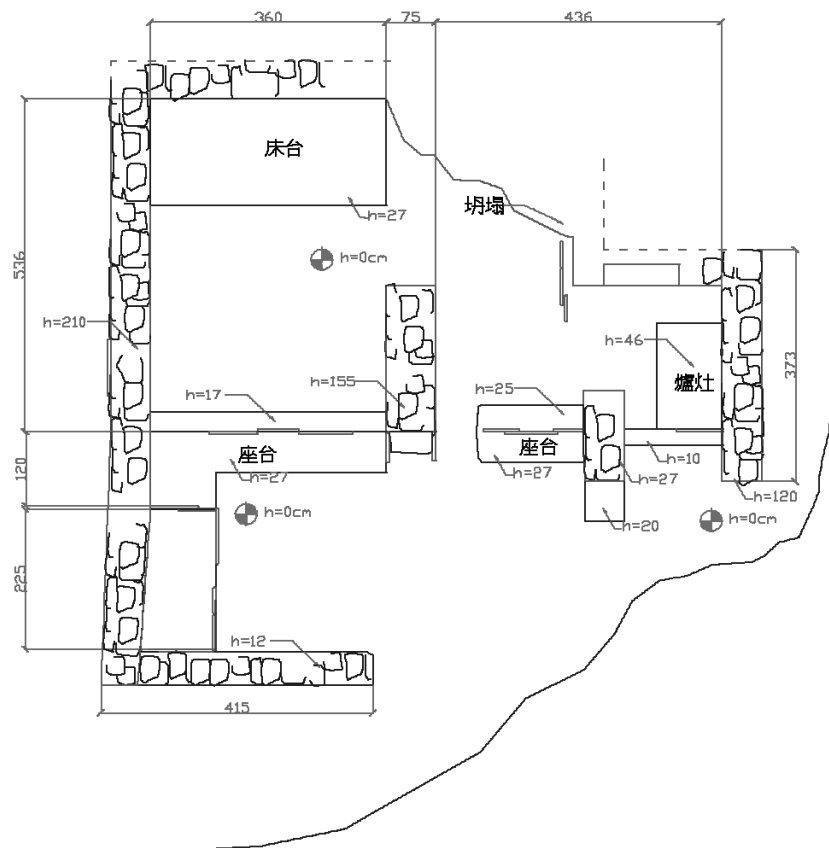
【圖 3-2-6】張杉其（編號 109）家屋及前庭配置圖 22
