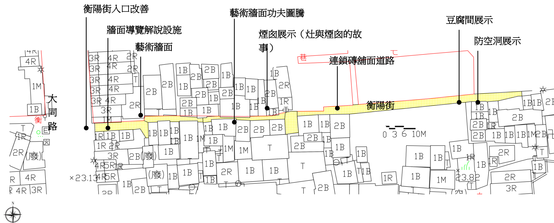
圖 5-1-17 傳統豆腐老街環境改善工程配置圖（單位M）
