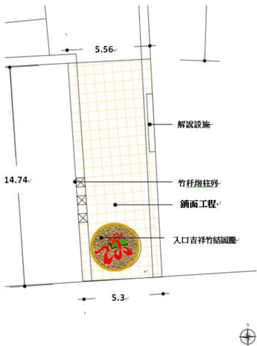
圖 5-1-8 河婆客家生活環境入口工程平面配置圖（單位M）
