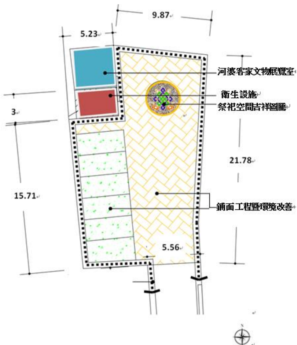
圖 5-1-5 擲老爺祭祀空間改善工程平面配置圖（單位M）
